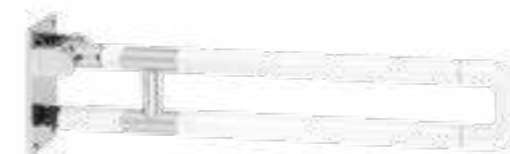
AC-332 BARRA DOBLE FRONTAL ABATIBLE 122€ + IVA Acero Inox 304 + ABS Cromado Desplegada: 8 x 20 x 62 cm Plegada: 8 x 73 x 14,5 / Ø 35 mm
