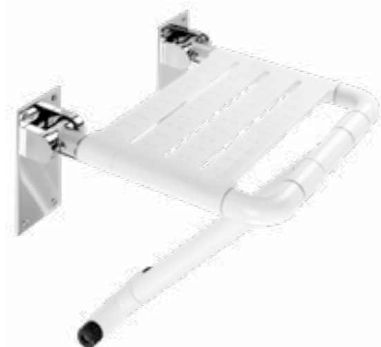
AC-325 ASIENTO DE DUCHA ABATIBLE 232€ + IVA MAX. 250 KG Acero Inox 304 + ABS Cromado Desplegado: 39,5 x 47 x 38 cm Plegado: 39,5 x 56 x 11 cm Barra de apoyo de 52,5 cm
