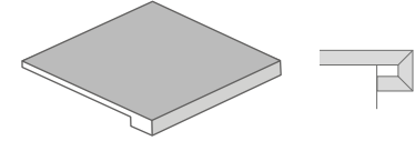
Peldaño Doble Gradone Fango Bianco 30x90 cm. 11 13/16 "x35 7/16 " P3090
