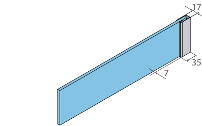
Cotas en mm.
