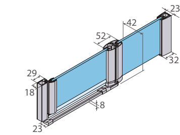
Cotas en mm.
