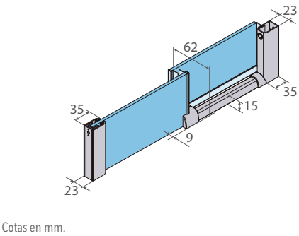
Cotas en mm.
