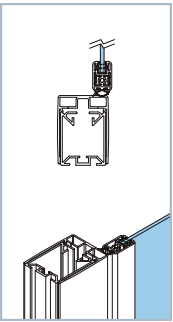
REFERENCIADO: Perfil con cierre magnético. Apertura interior.
