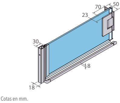
Cotas en mm.
