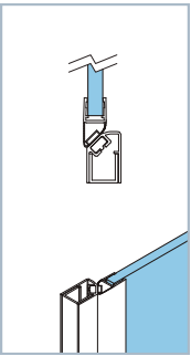
Perfil con cierre magnético. Apertura exterior.
