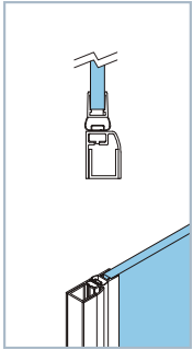
REFERENCIADO: Perfil con cierre magnético. Apertura Interior o exterior.
