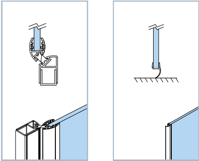
REFERENCIADO: Perfil con cierre magnético. Apertura exterior. Cierre contacto. Apertura interior y exterior.
