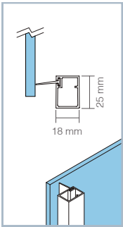
OPCIONAL: Perfil con cierre contacto.
