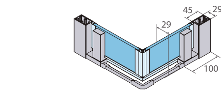
Cotas en mm.
