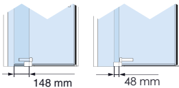
SOLAPE KE-216. Sin compensar 148 mm y compensada al máximo 48 mm.
