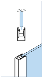
Perfil con cierre junquillo.
