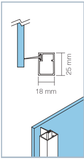
REFERENCIADO: Perfil con cierre contacto.
