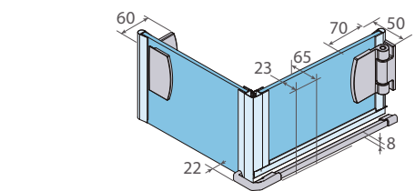
Cotas en mm.
