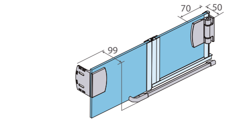
Cotas en mm.
