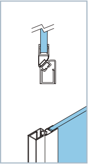
Perfil con cierre magnético. Apertura exterior.
