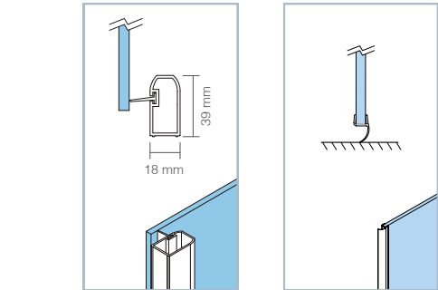
REFERENCIADO: Perfil con cierre contacto. Cierre contacto.
