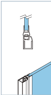
Perfil con cierre magnético. Apertura Interior o exterior.
