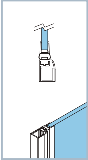
Perfil con cierre magnético.
