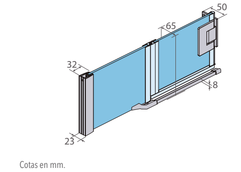
Cotas en mm.
