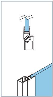
Perfil con cierre magnético. Apertura exterior.
