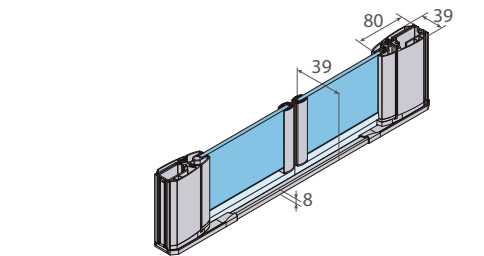
Cotas en mm.
