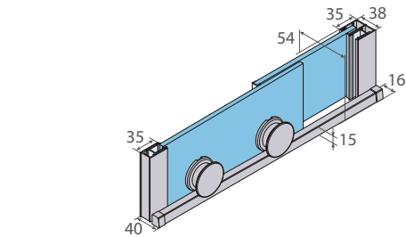
Cotas en mm.
