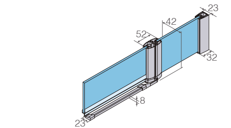
Cotas en mm.
