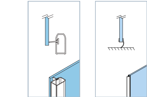
Perfil con cierre contacto. Cierre contacto.
