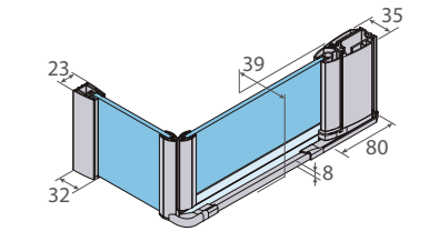
Cotas en mm.
