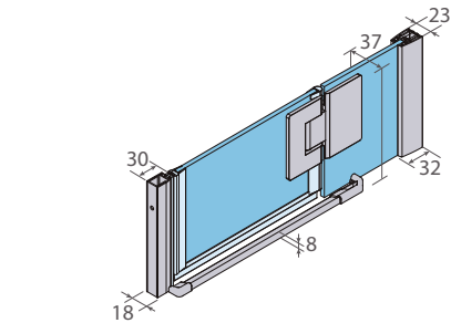
Cotas en mm.
