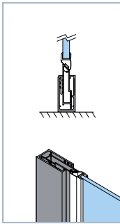
Perfil con cierre magnético. Apertura Interior o exterior.
