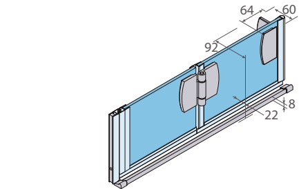
Cotas en mm.
