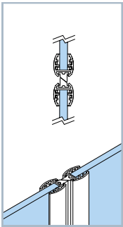
REFERENCIADO: Perfil con cierre magnético. Apertura exterior.
