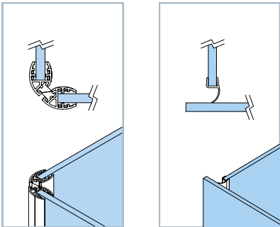
Perfil con cierre magnético. Apertura exterior. Cierre contacto. Apertura interior y exterior.
